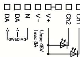
Anschlussplan Dose 8A
