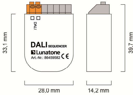
Abmessungen Dose
