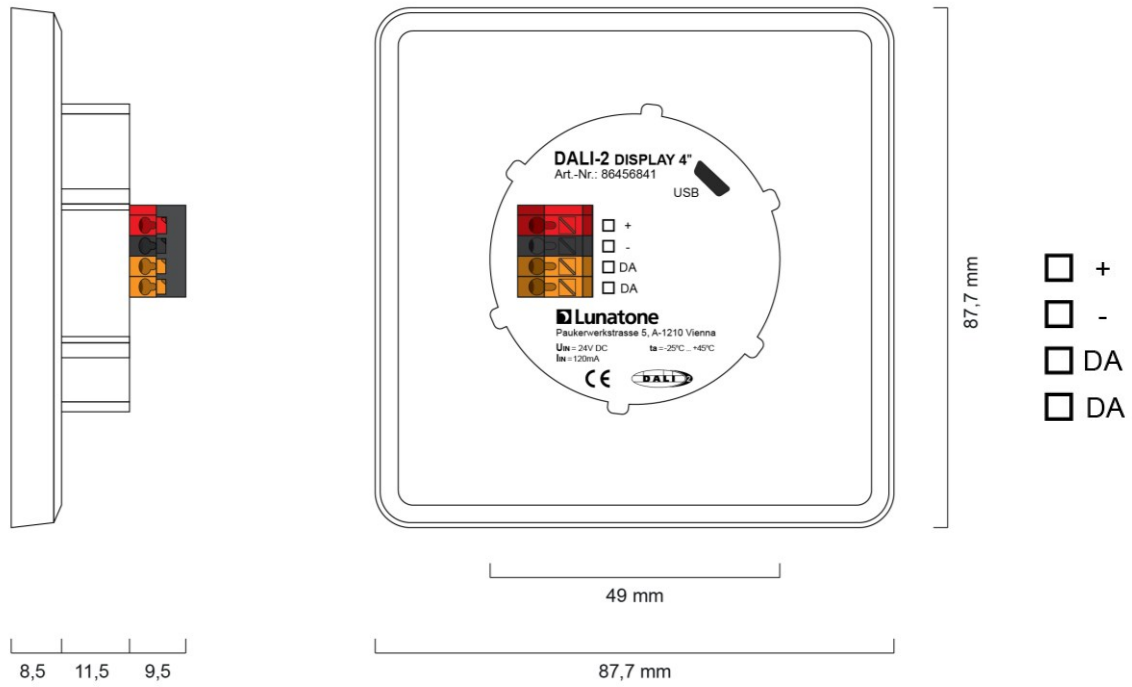
Dimensions Art.Nr.: 86456841-...
